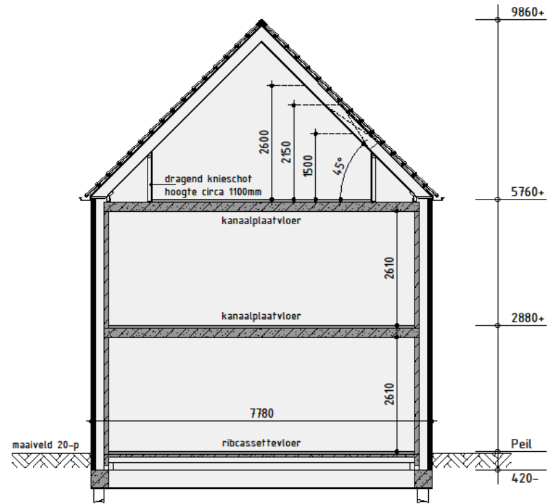
Principe doorsnede A-A
